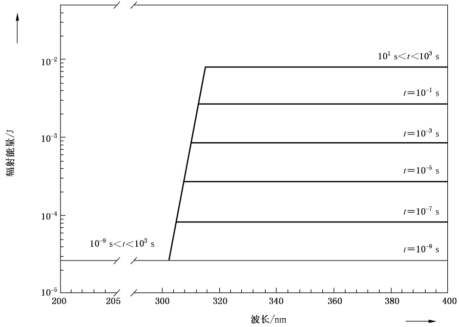
图 B.3 对选定发射持续时间 10^{-9} \text{ s} \sim 10^3 \text{ s} 的 1 类紫外激光产品的 AEL 值
